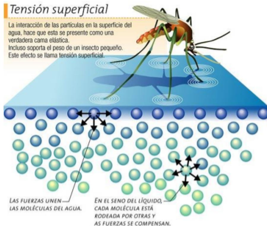
Fig. 7. Tensión superficial.
